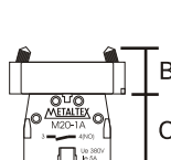
Dimensões dos blocos Block dimensions
