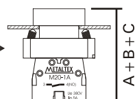
Dimensões do atuador + blocos Button + Blocks dimensions
